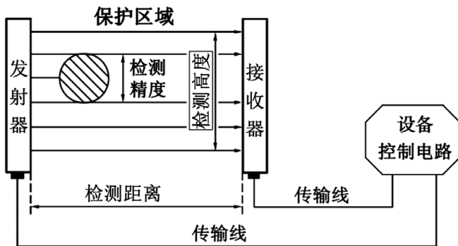
图1 安全光栅工作示意图
