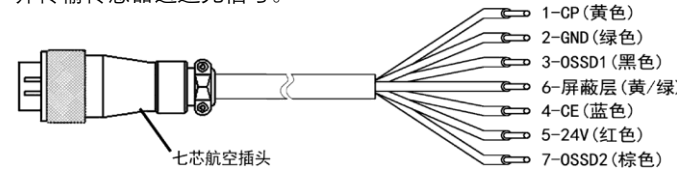
图1.2 LA4型单端传输线
