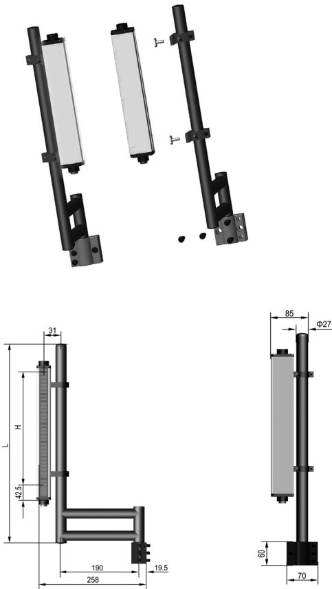
6.4 双臂支架侧装 –T 型槽安装方式（SCT）
