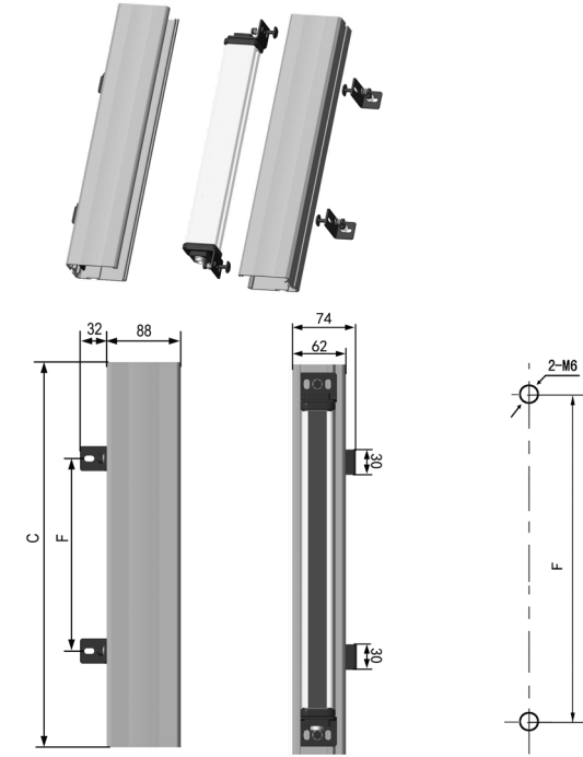
6.7 防护罩侧装方式（FC）
