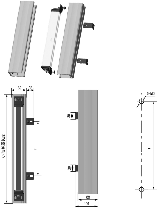
6.6 防护罩正装方式（FZ）
