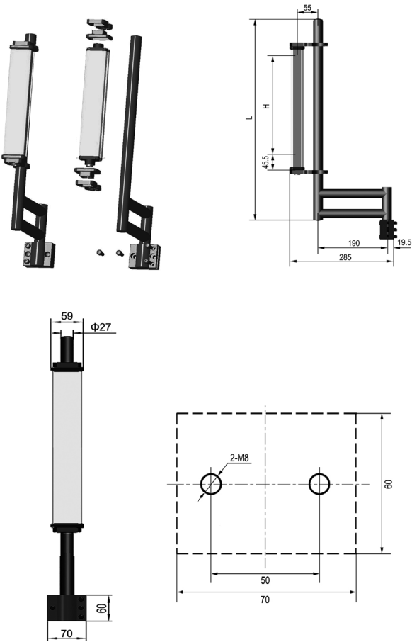
6.3 双臂支架侧装 – 带减振器安装方式（SCJ）
